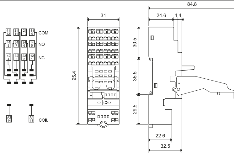
Fassung + Kammbrücke
