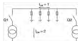
Doppeleinspeisung links/rechts
