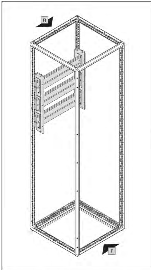
Bestückung Sammelschienenhalter 50 x 10 Rückbereich
