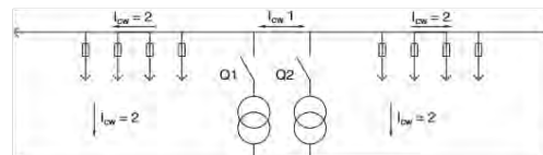
Doppelmitteneinspeisung
