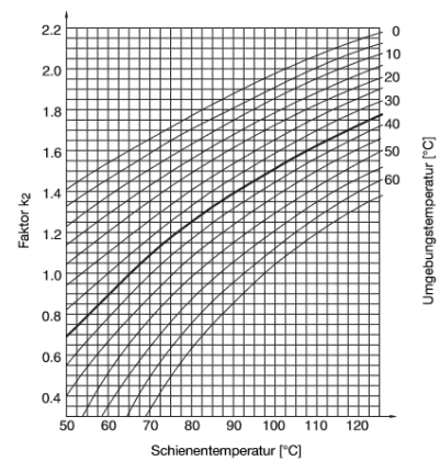
Korrekturfaktordiagramm nach DIN 43 671
