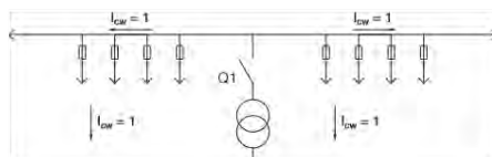
Mitteneinspeisung
