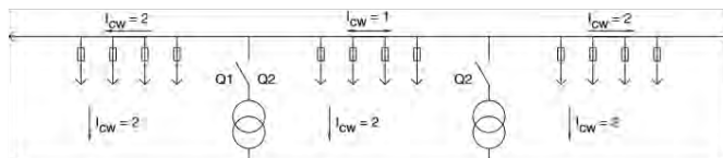
Doppeleinspeisung
