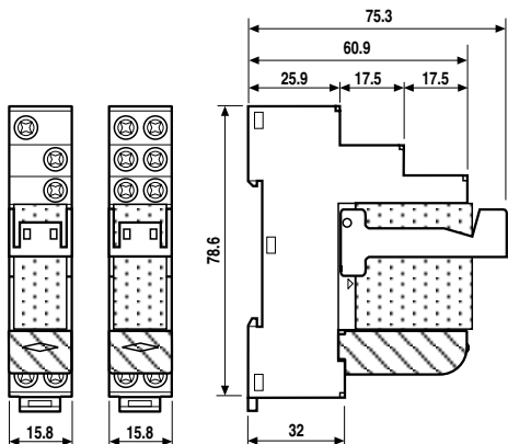
48.31 48.52 / 48.61 / 48.62 Schraubklemmen
